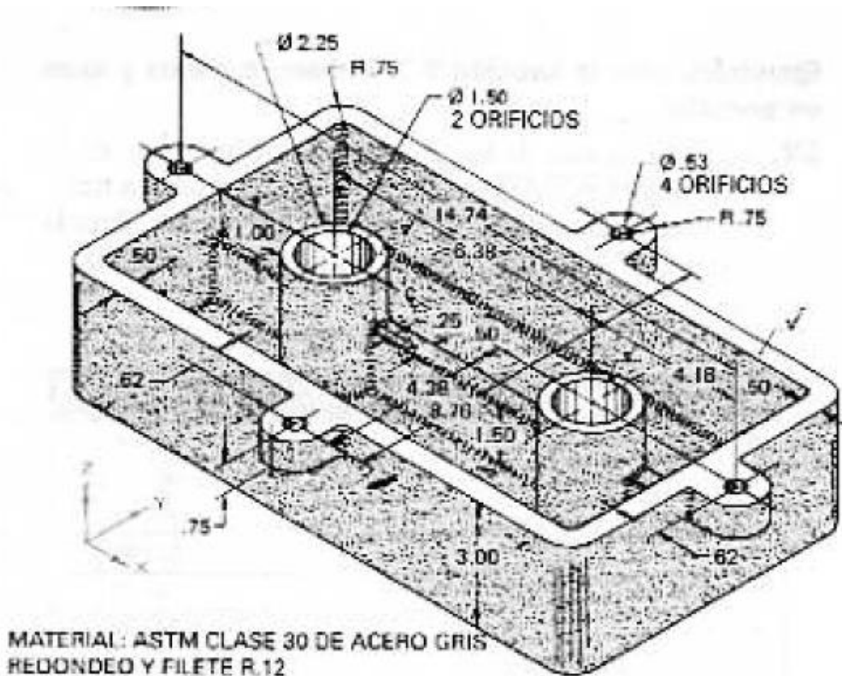
Figura 1. Base de columna de dos postes.
